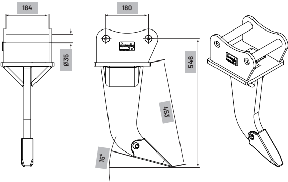
76456-Dent de déroctage M10 6-10 t Pointe de la dent : dent de chargeur Bofors 6500.54
