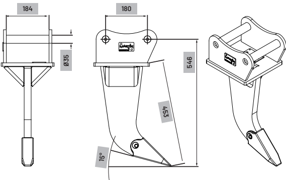
76456-Aufreibzahn M10 6-10to Zahnspitze: Hülsenzahn Bofors 6500.54
